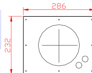
KUVUN KATTOKIINNIKKEEN MITOITUS, LIITÄNTÄKANAVAN KOKO Ø125
